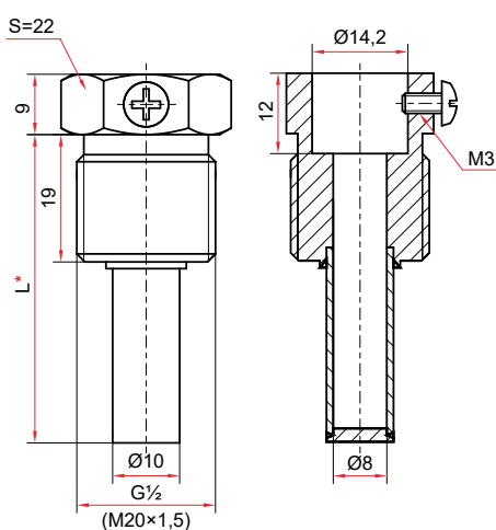
Гильза для термометров БТ серии 211
